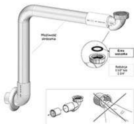
PUM - zestaw odpływowy z rurą sztywną 8075536 - biały 8075537 - chrom
