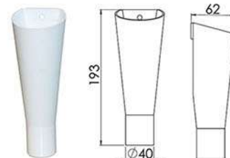
PUM - syfon suchy do odprowadzania kondensatu 8077178
