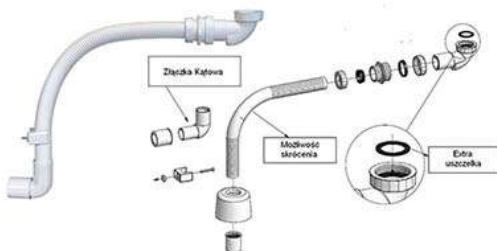
PUM - zestaw odpływowy z rurą karbowaną 8075628
